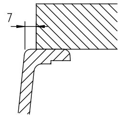
Ausschnitt Unterbau 1:20
