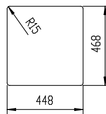
Ausschnitt Unterbau 1:20
